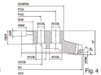
Čeono i kutno glodanje
